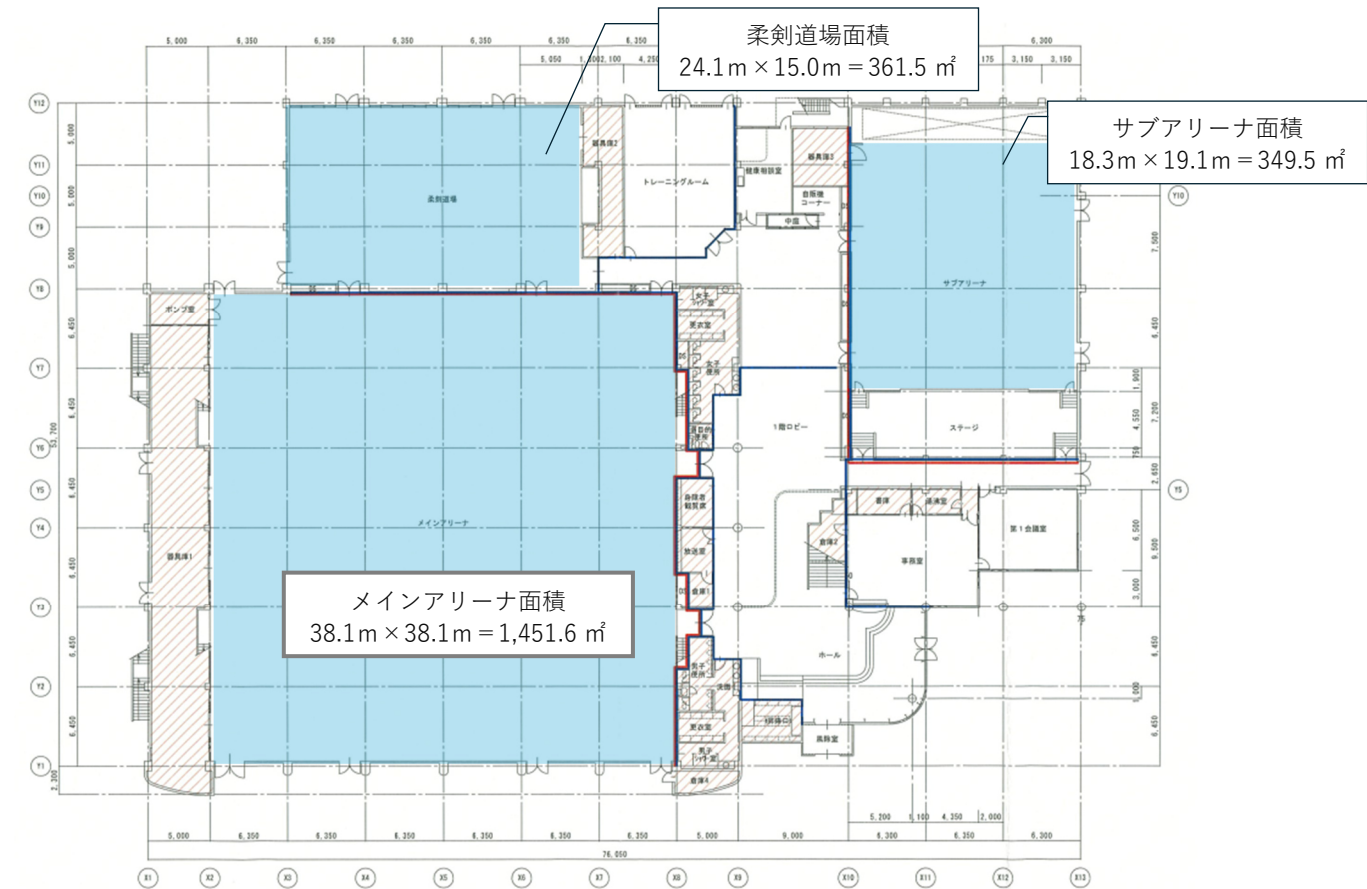
総合体育館 1階平面図
