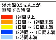
浸水継続時間分布図
