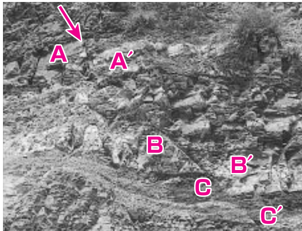
師崎層群の断層 片名・蛭子
