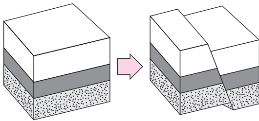
断層のでき方を示す模式図
