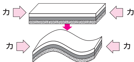
褶曲のでき方を示す模式図
